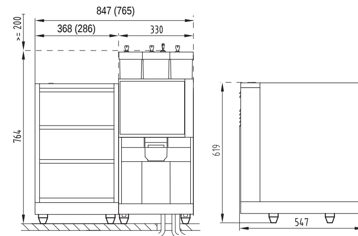
Maschinenfront
