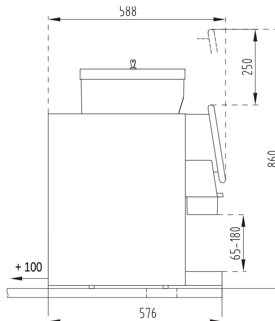
Seitenansicht Maschine
