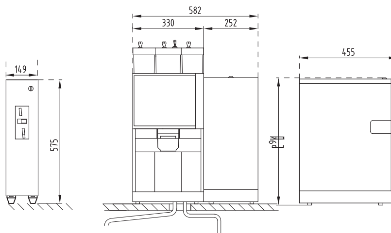
Maschinenfront
