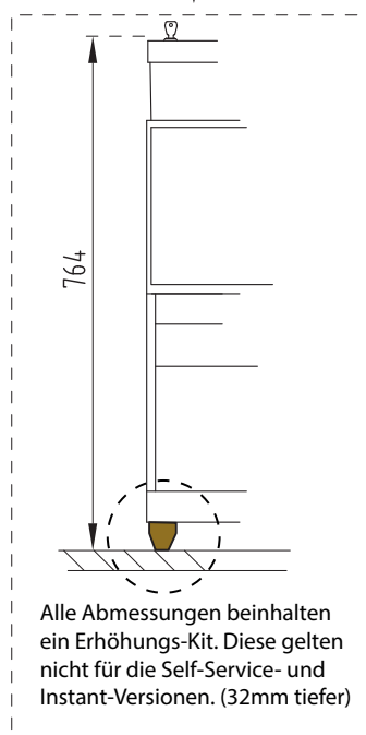
Maschinenfront
