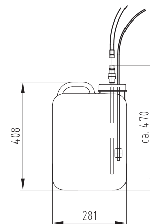
Trinkwassertank 16L
