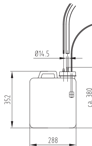
Schmutzwassertank 13L
