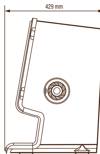
Seitenriß
