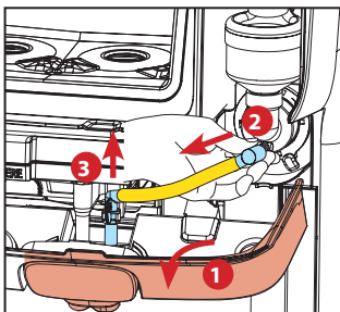
Abbildung 2 – Das Wasserauffbereitungsfach (1) öffnen, den Auslassanschluss vom Mischbecher abziehen (2) und den Auslass vom Clip abziehen (3).
