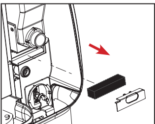
Abbildung 7 Den Kondensatabscheiderfilter samt Abdeckung entfernen.
