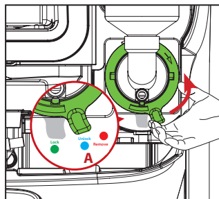
Abbildung 3 – Die Verriegelung der Montageplatte gegen den Uhrzeigersinn in die entriegelte Position (A) drehen.
