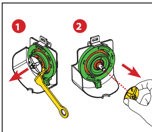
Abbildung 5 – Zum Entfernen des Aufschäumers das mitgelieferte Werkzeug verwenden. Das Werkzeug hinter dem Aufschäumer ansetzen. Das Werkzeug am Griff leicht nach innen drücken, um den Aufschäumer zu lösen (1). Den Aufschäumer gerade herausziehen (2).
