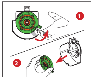
Abbildung 6 Die Montageplatte gegen den Uhrzeigersinn über die Position „Entfernen“ hinaus drehen, bis sie sich nicht mehr weiterdrehen lässt (1). Die Platte gerade herausziehen (2).
